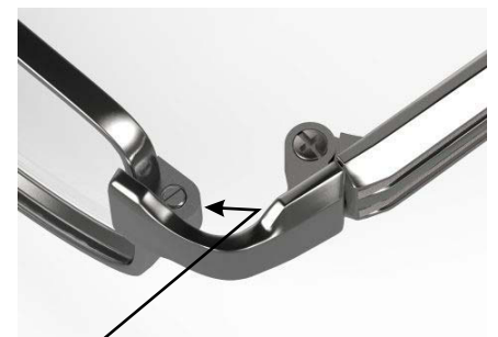
バックスクリューネジ (スリ割り加工付き)
